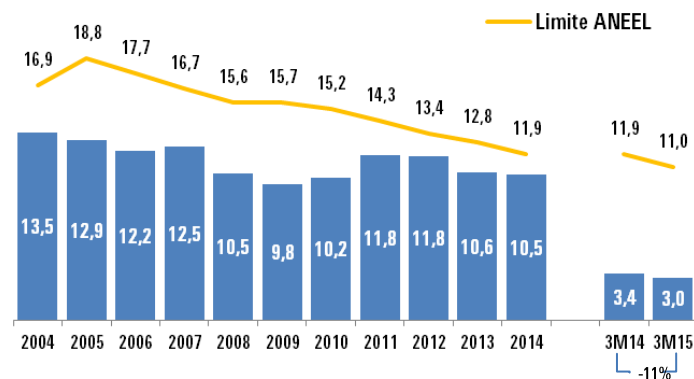
FEC - FREQUÊNCIA EQUIVALENTE POR CONSUMIDOR (número de vezes)
