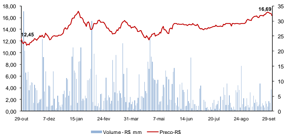
CTIP3 Preço (R$) vs. Volume (R$ mm) (29/10/2009 - 30/09/2010)
